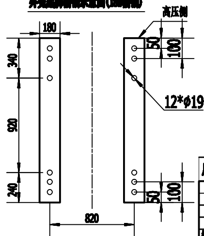
外壳内部结构示意图(100mm比例)
