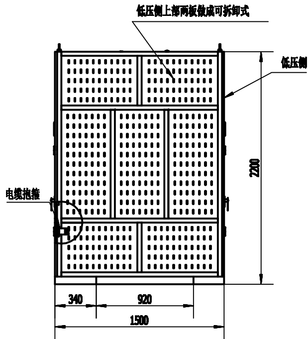
外壳内部结构示意图(100mm比例)
